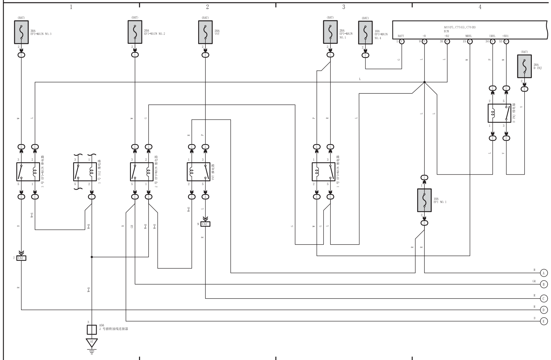
电子控制变速器和 A/T 档位指示器 (A25A-FKS)、发动机控制 (A25A-FKS)
